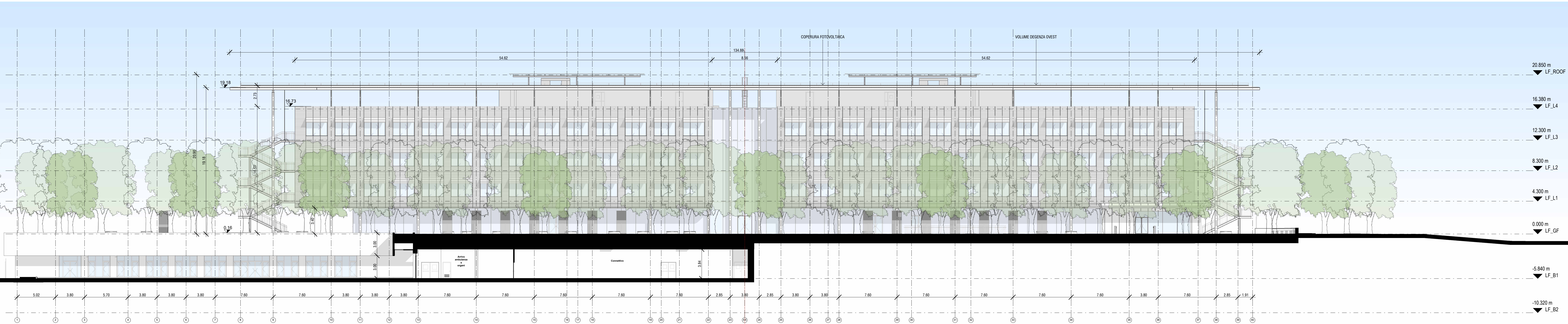
Prospetto Ovest scala - 1 : 200
