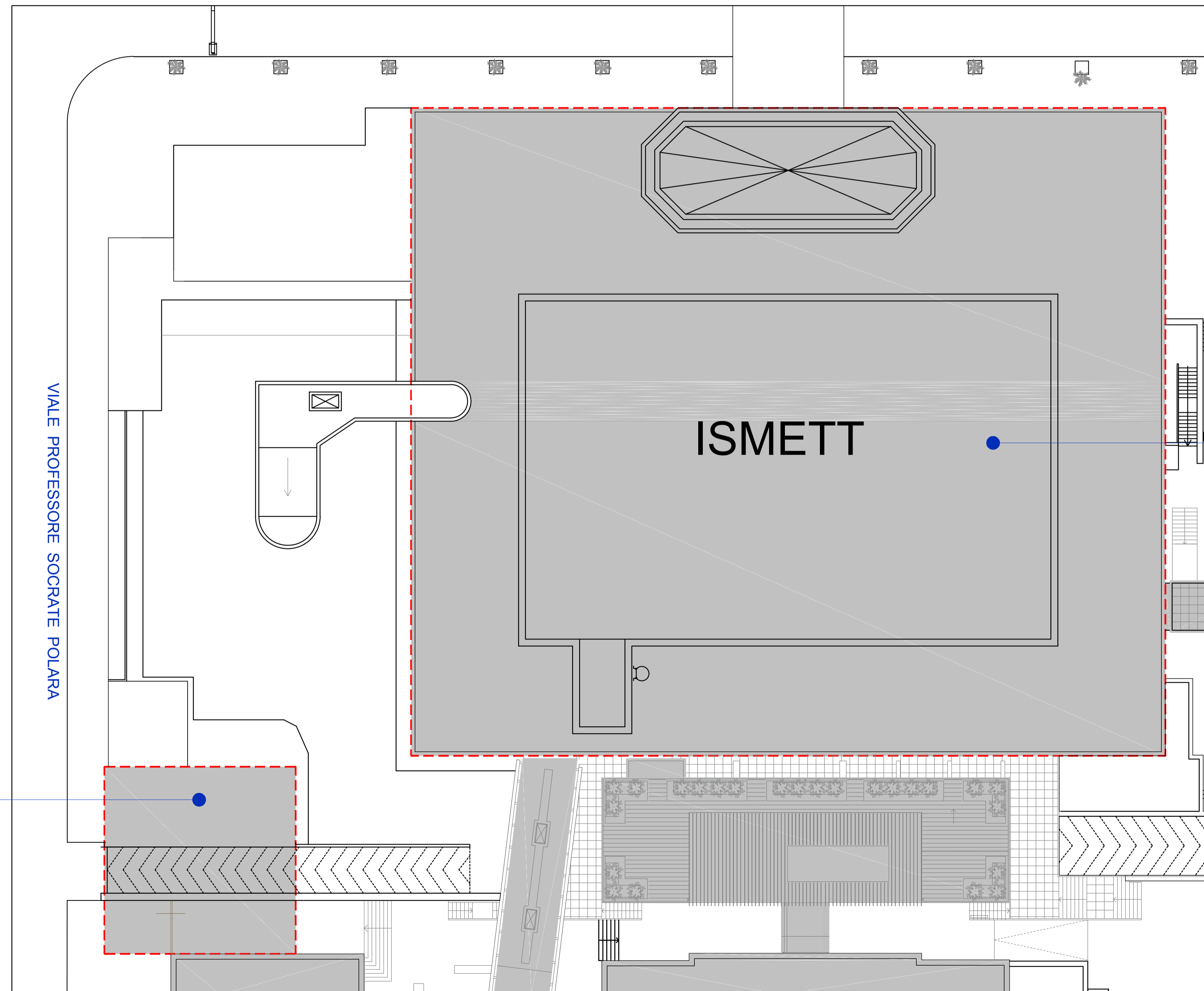
Planimetria generale 1:200
